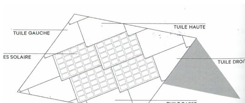
Tuiles solaires Sunstyle, source : d'a n°286 dec 2021, De la tuile solaire à l'enveloppe du bâtiment: «le moment est venu» B.Joly.
